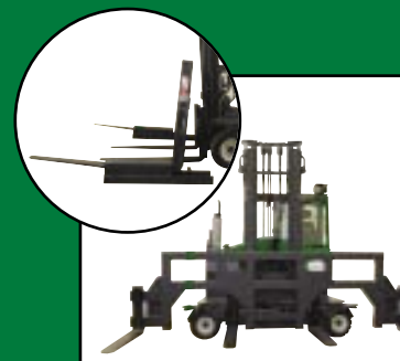
Aufnehmbarer Langgutabelträger mit 4 Gabelzinken
