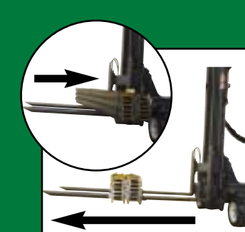
Teleskopgabeln (eingefahren / ausgefahren)
